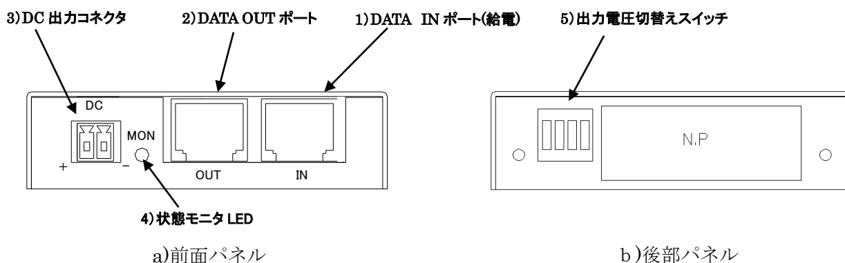
図1 各部の配置
